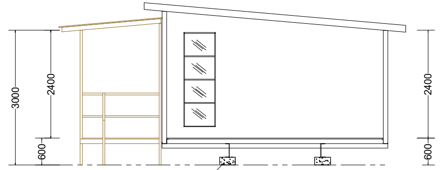
Right Elevation
